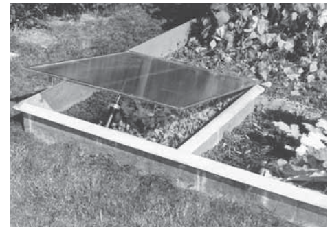
In der Ecke eingebautes Treibbeet, Befestigung mit 2 Winkeln, Lüftungsautomat
